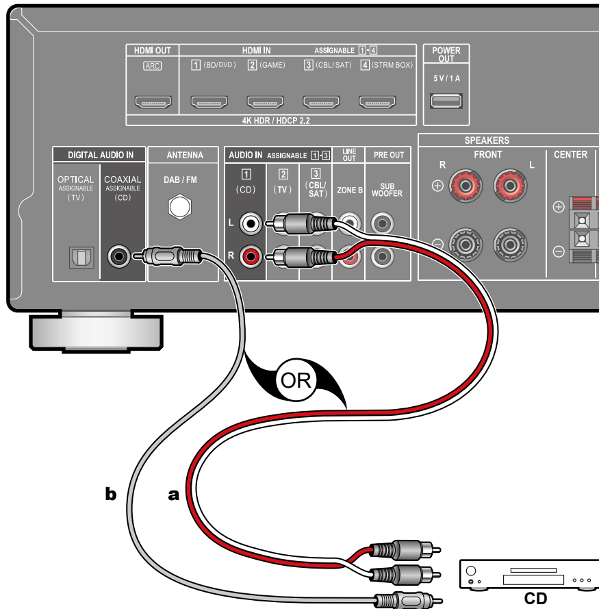
a Cavo audio analogico, b Cavo digitale coassiale
