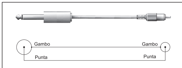
Fig. 5.2: cavo adattatore mono
