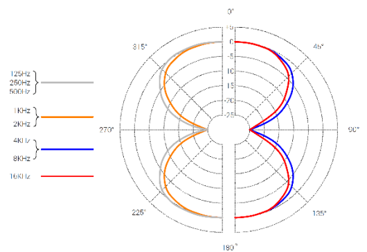
Diagramma polare
